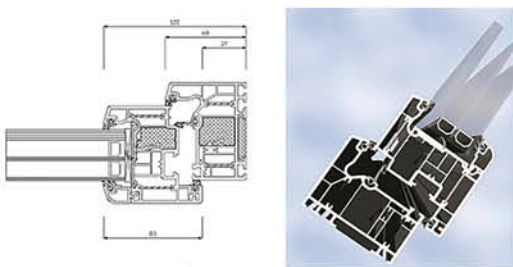
Eindrucksvoll ist die maßstabsgetreue Darstellung der Elemente in der Schnittansicht.
